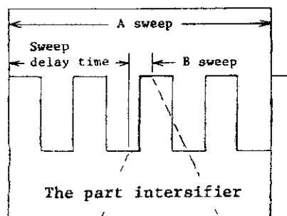
HORIZ DISPLAY A INTEN
